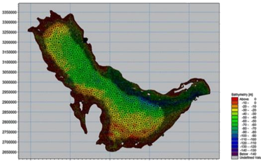
نمونه ای از مدل سازی جریان توسط نرم افزار مایک
