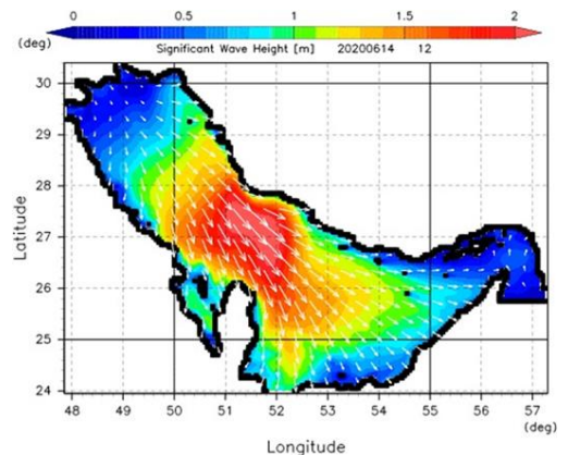
نمونه ای از مدل سازی موج با استفاده از خروجی نرم افزارهای Matlab و Mike21
